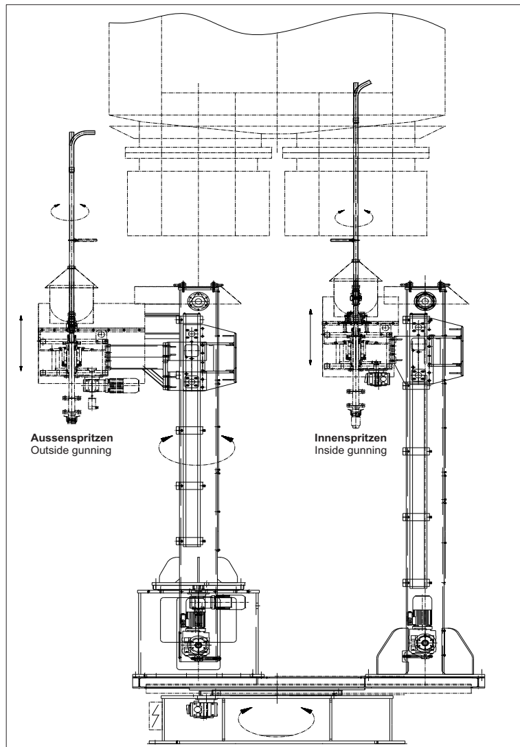
Manipulator TR 54 mit 6 Freiheitsgraden Manipulator TR 54 with 6 degrees of freedom
